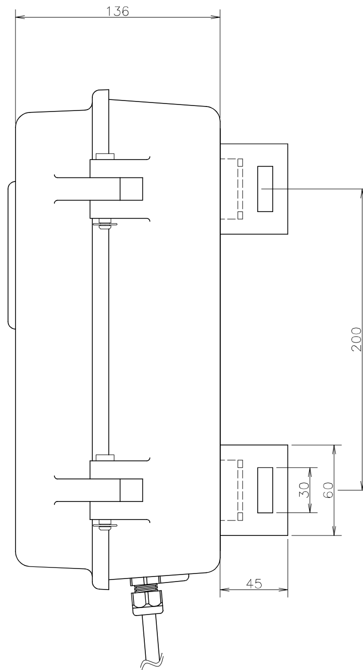
図面名称 絶縁破壊検知器 外形図
