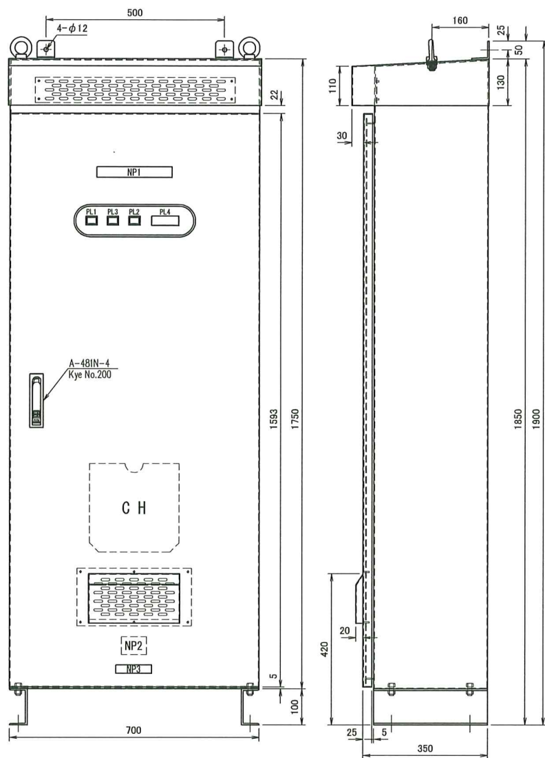
外形図
