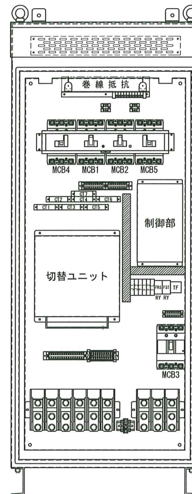
内部配置図
