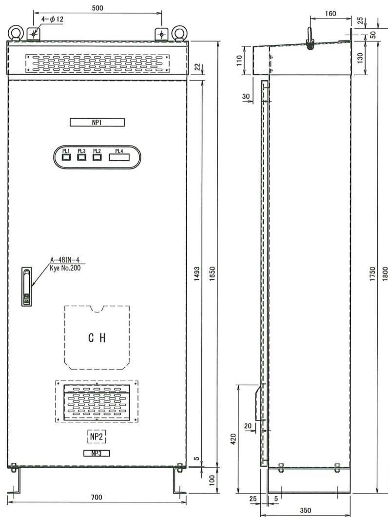
外形図
