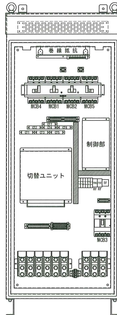
内部配置図
