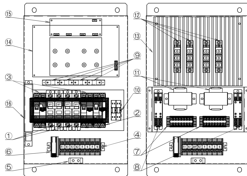
20/30A入出力端子台(M5 最大16mm 2 端子幅12.2mm)
