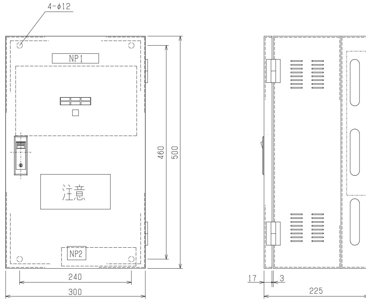
外形図
