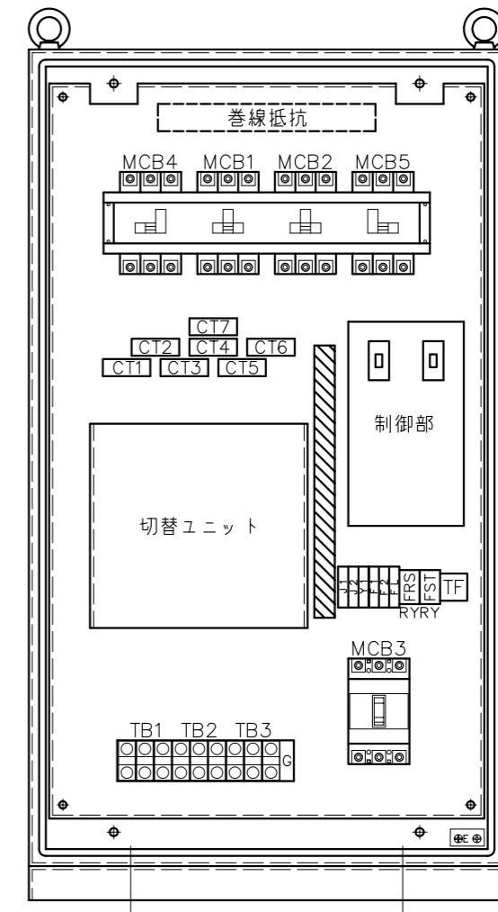
内部配置図
