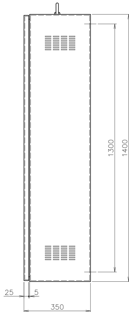
外形図
