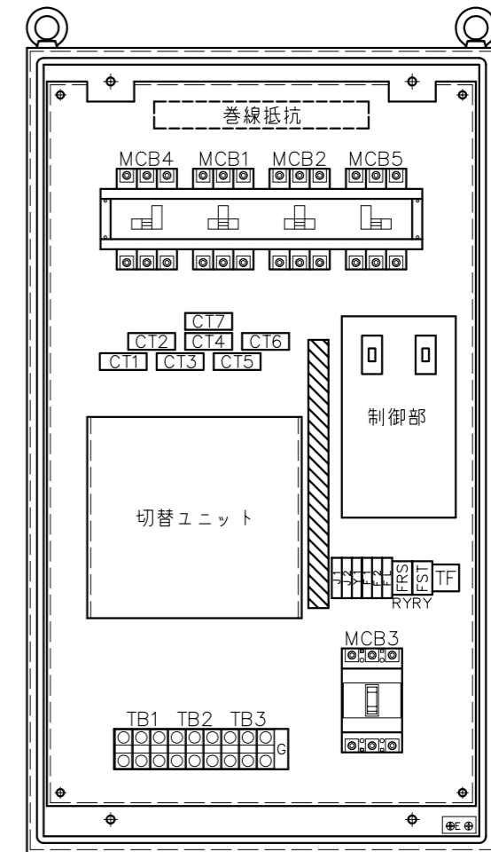
内部配置図
