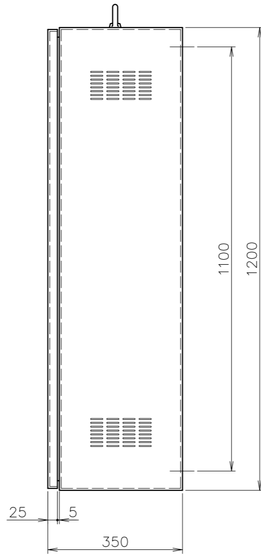
外形図
