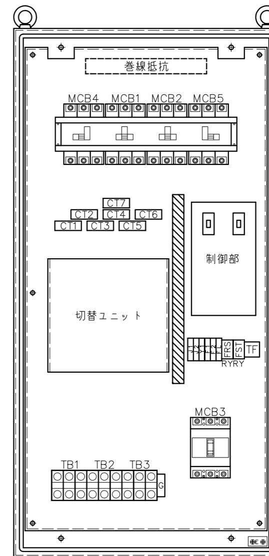
内部配置図
