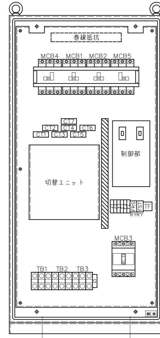
内部配置図
