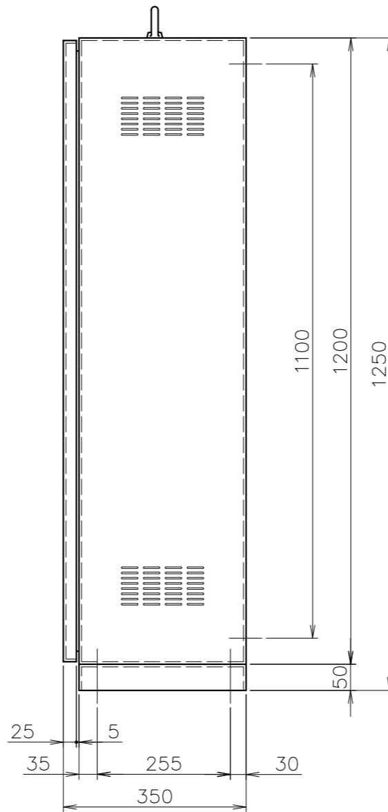
外形図
